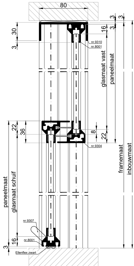
VERTECALE DOORSNEDE type VSL-4A
