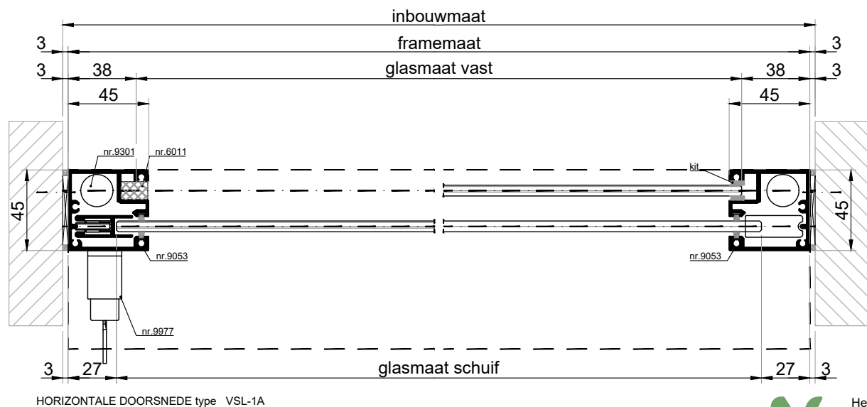
HORIZONTALE DOORSNEDE type VSL-1A
