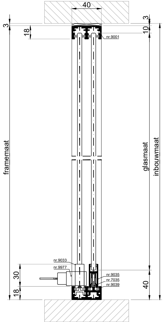
VERTICALE DOORSNEDE type HSL-4A
