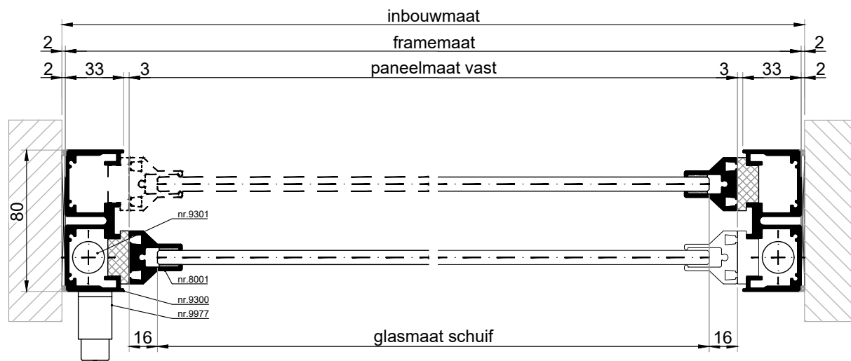
HORizontale DOORSNEDE type VSL-4A
