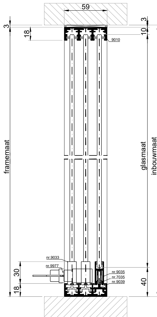
VERTICALE DOORSNEDE type HSL-2G
