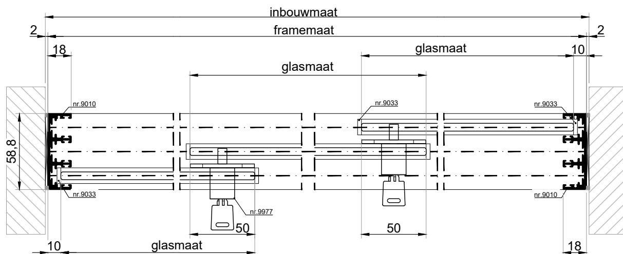
HORIZONTALE DOORSNEDE type HSL-2G
