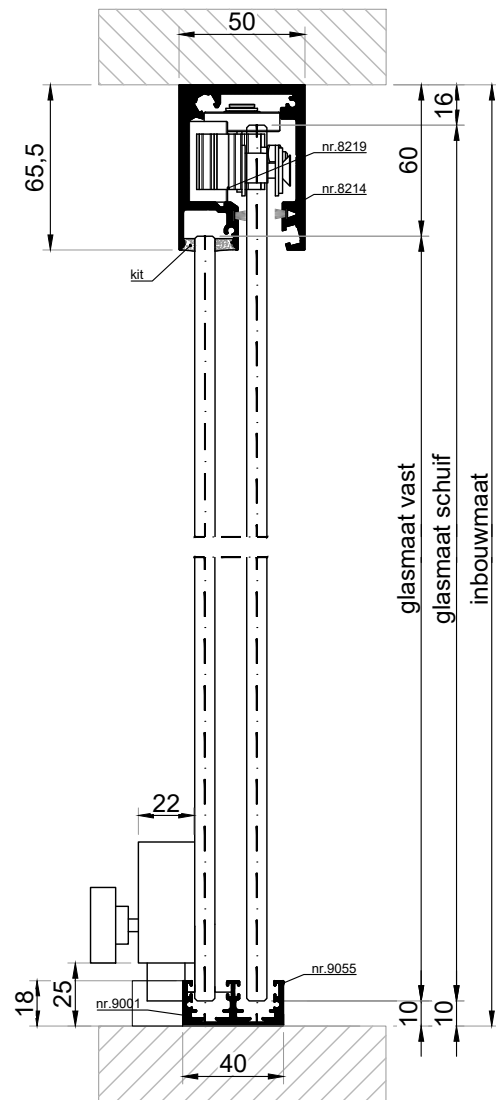
VERTICALE DOORSNEDE type HSL-10B
