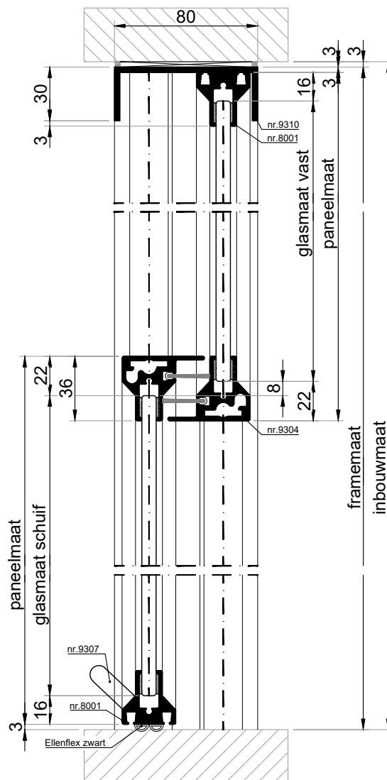
VERTICALE DOORSNEDE type VSL-4A
