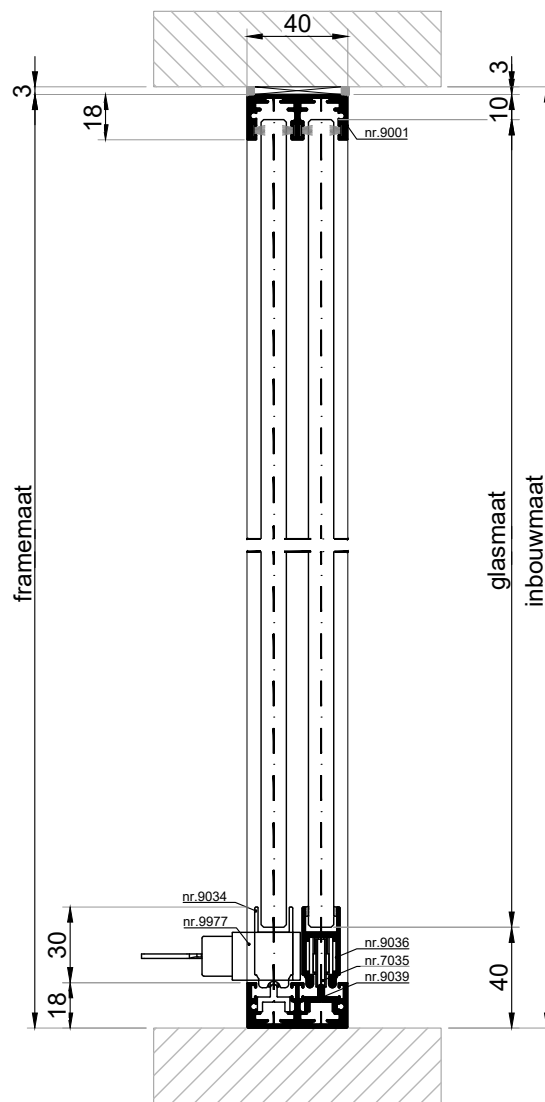
VERTICALE DOORSNEDE type HSL-3A
