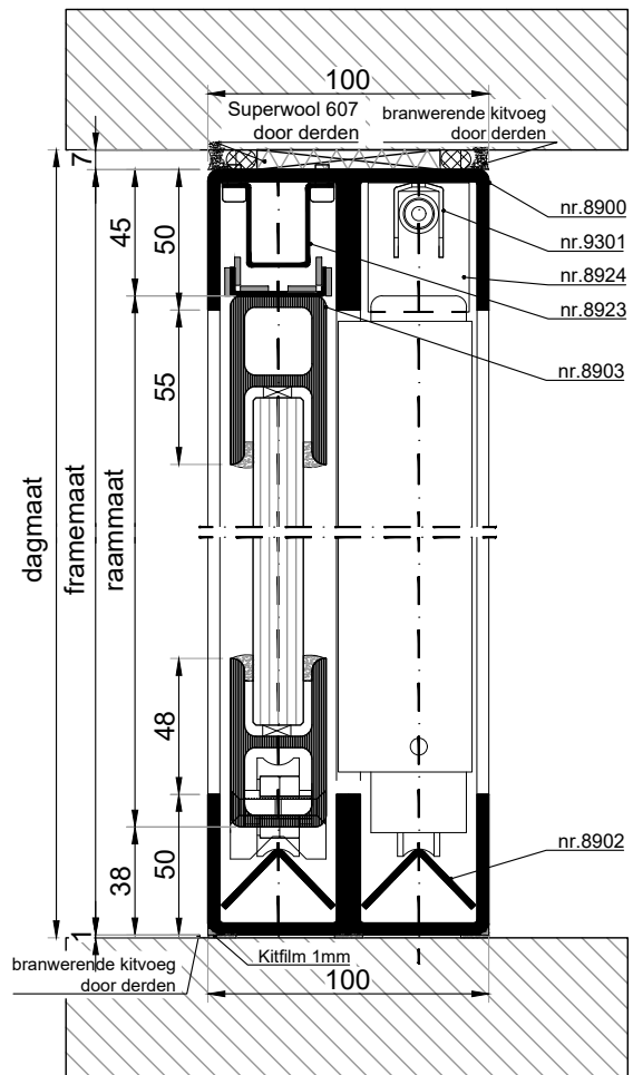
VERTICALE DOORSNEDE type MHSL-1E
