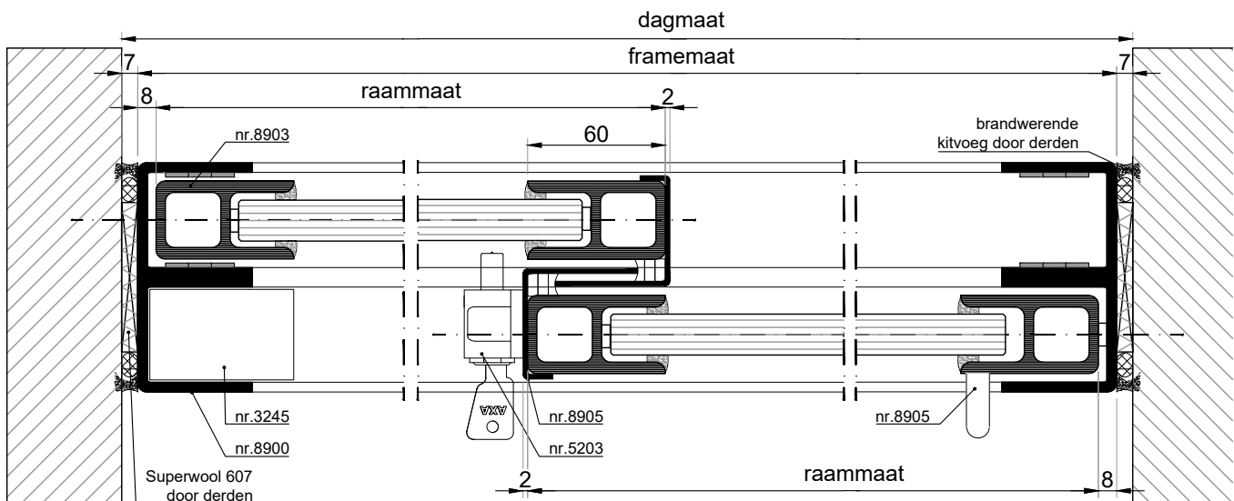
HORIZONTALE DOORSNEDE type MHSL-1B
