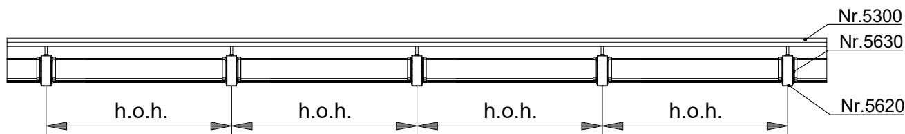
VERTICALE DOORSNEDE type TLH-1A
