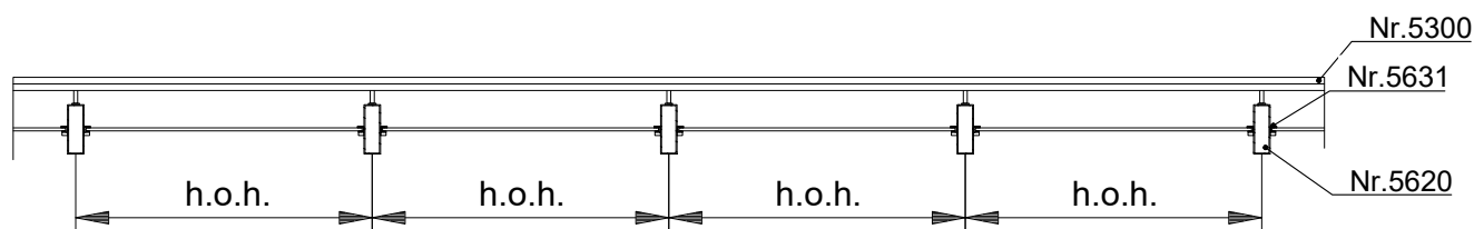
VERTICALE DOORSNEDE type TLH-1E
