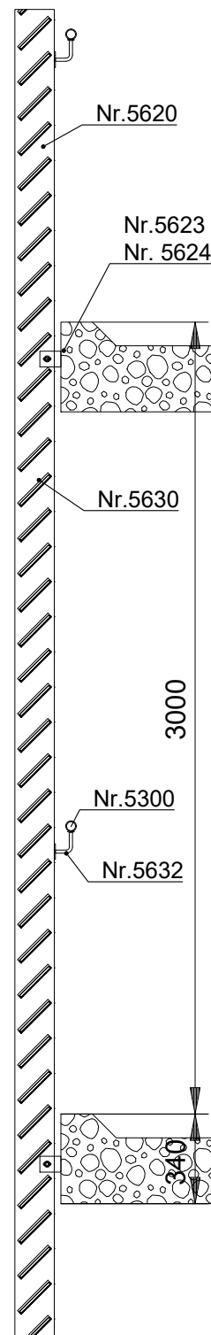
VERTICALE DOORSNEDE type TLH-1A
