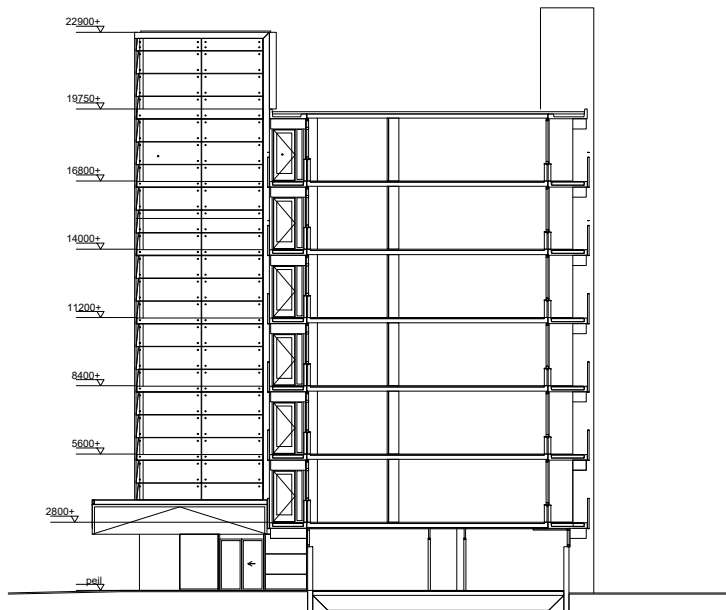
ZIJAAANZICHT GEVELFRAGMENT
