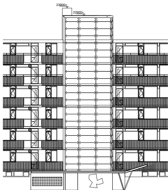
VOORAANZICHT GEVELFRAGMENT
