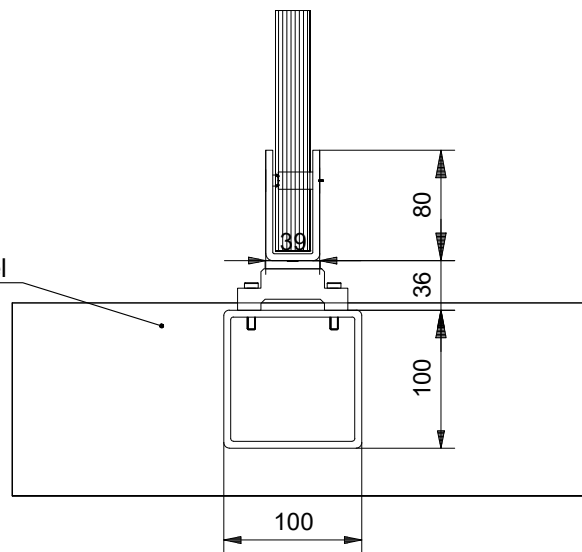
VERTICALE DOORSNEDE type TLVE-1
