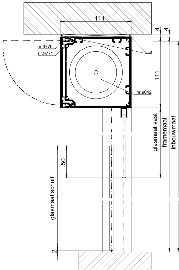
VERTICALE DOORSNEDE type EVSL-1A
