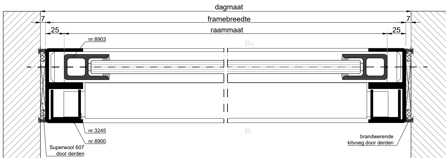
HORIZONTALE DOORSNEDE type AVSL-1A
