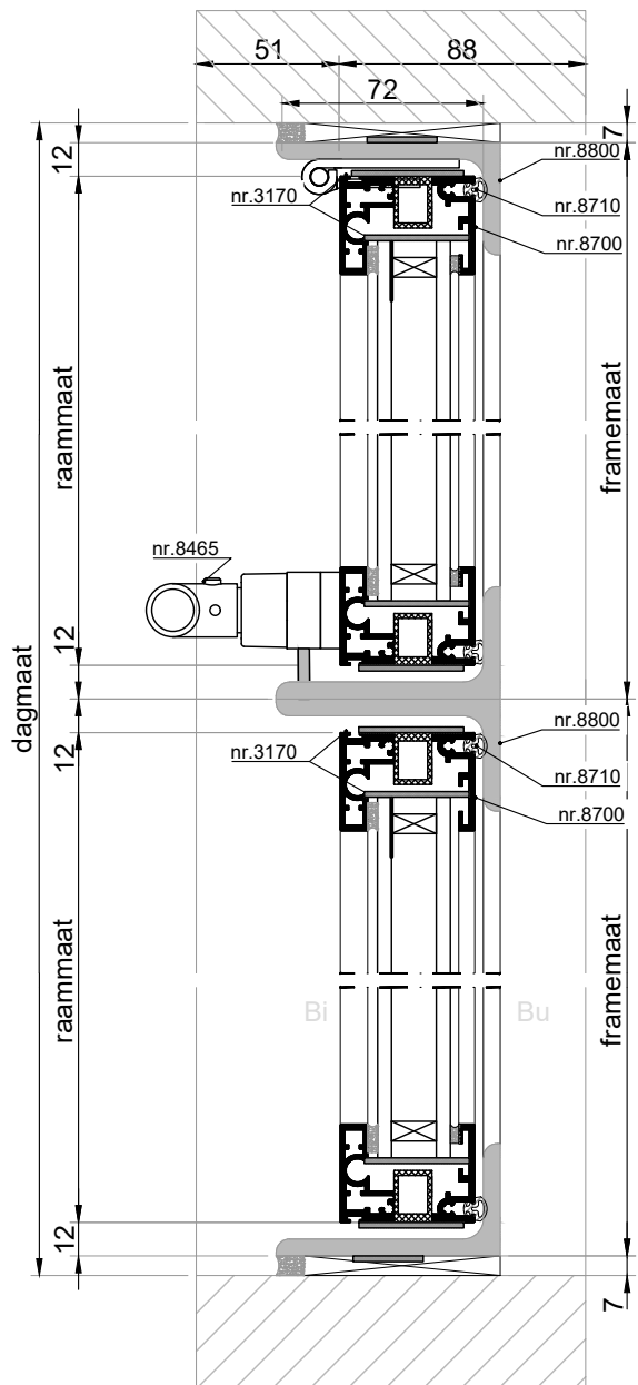
VERTICALE DOORSNEDE type AMC-3L
