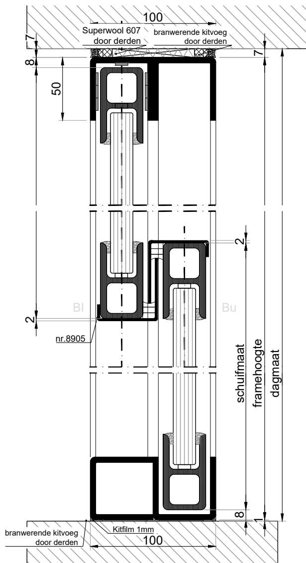
VERTICALE DOORSNEDE type AVSL-1A
