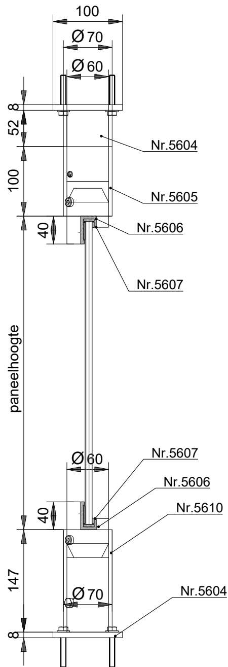
VERTICALE DOORSNEDE type TLV-2
