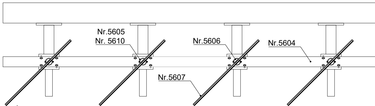
HORIZONTALE DOORSNEDE type TLV-2
