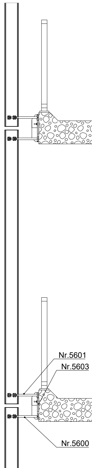
VERTICALE DOORSNEDE type TLV-1A
