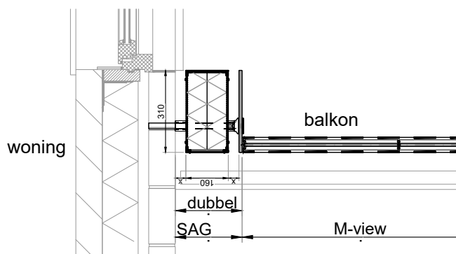
Type Box-10B-40x310 aan zijkant
