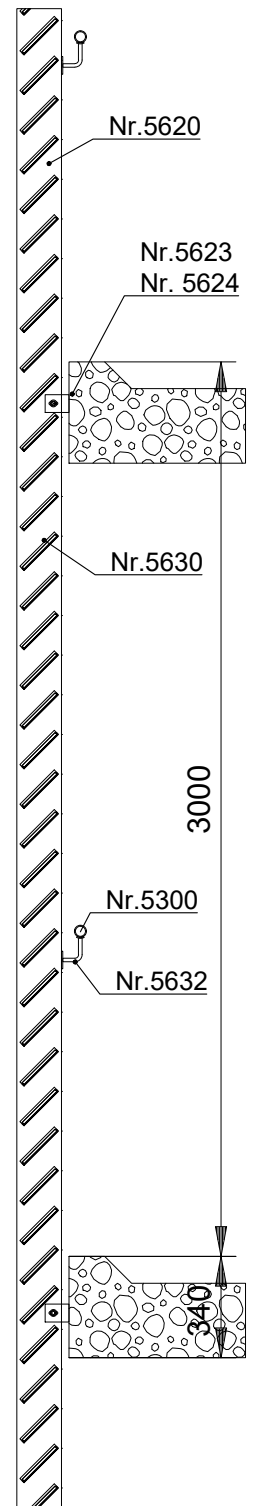
VERTICALE DOORSNEDE type TLH-1A
