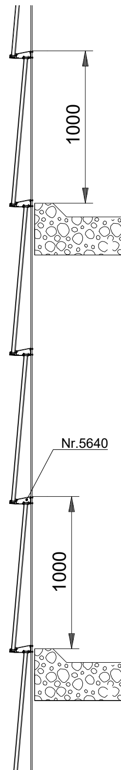
VERTICALE DOORSNEDE type TLH-2
