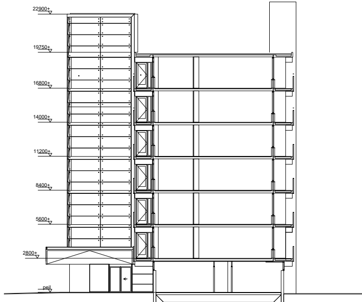
ZIJAAANZICHT GEVELFRAGMENT
