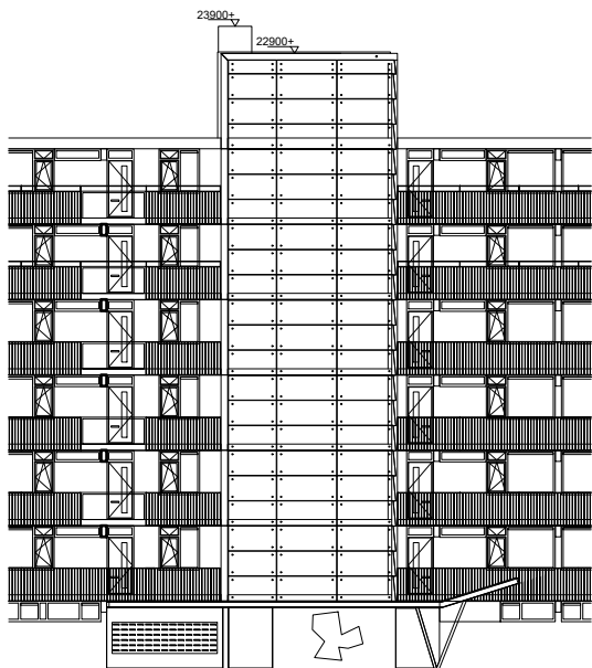
VOORAANZICHT GEVELFRAGMENT
