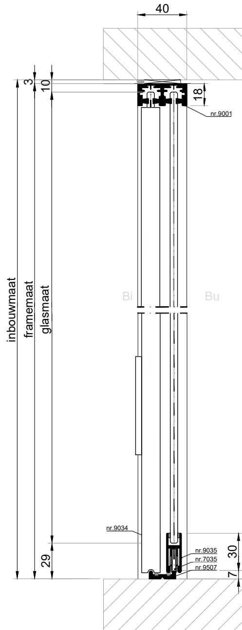
VERTICALE DOORSNEDE type HSV-2
