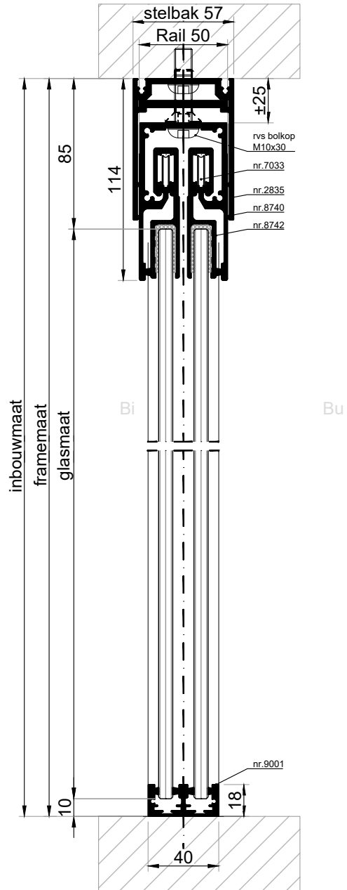
VERTICALE DOORSNEDE type ASH-3
