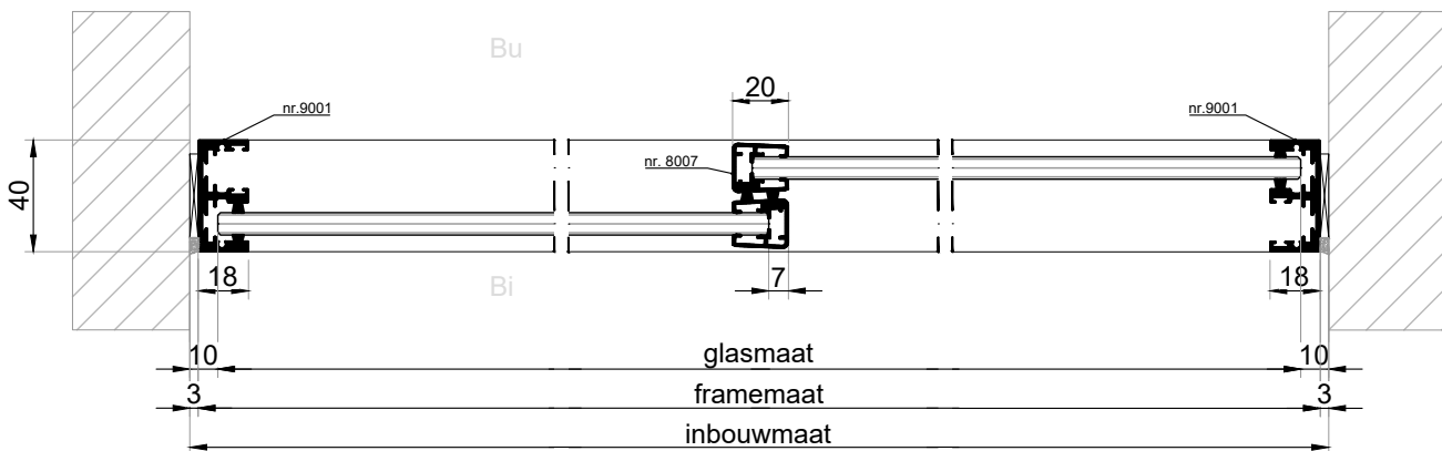
HORIZONTALE DOORSNEDE type ASH-2
