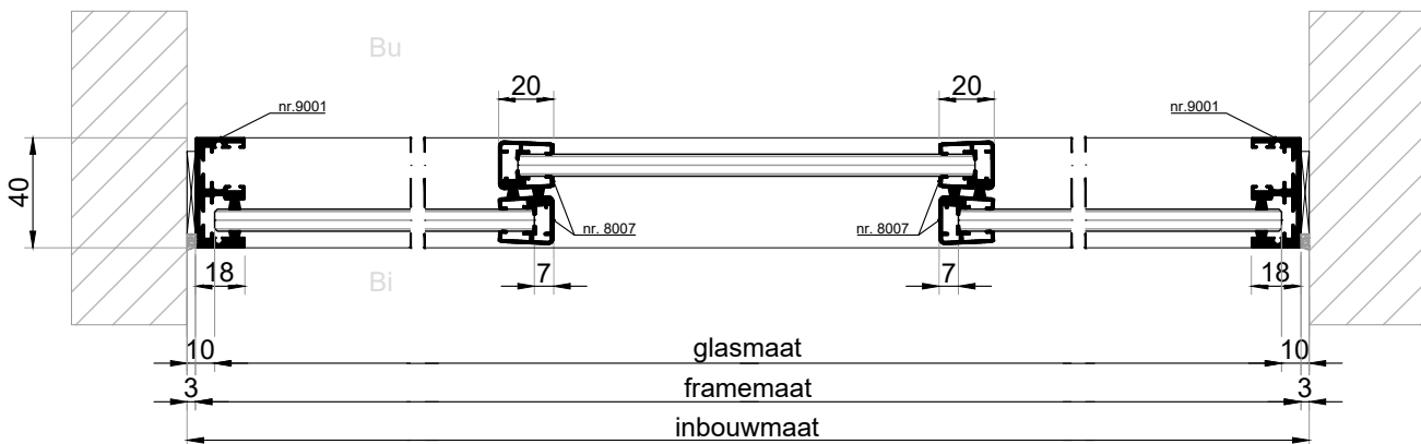
HORIZONTALE DOORSNEDE type ASH-3
