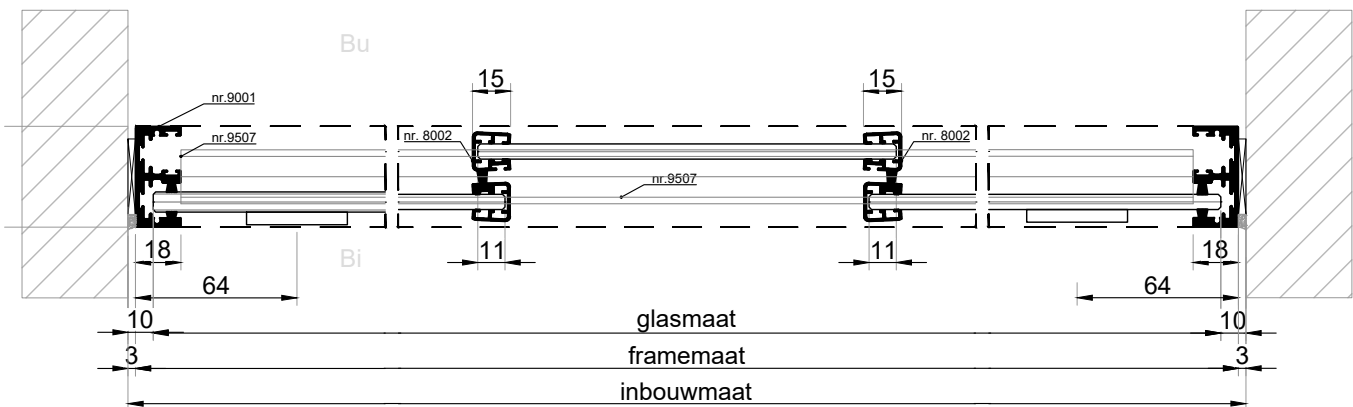
HORIZONTALE DOORSNEDE type HSV-3
