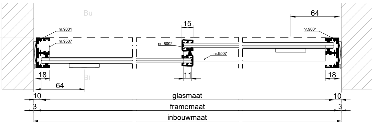
HORIZONTALE DOORSNEDE type HSV-2
