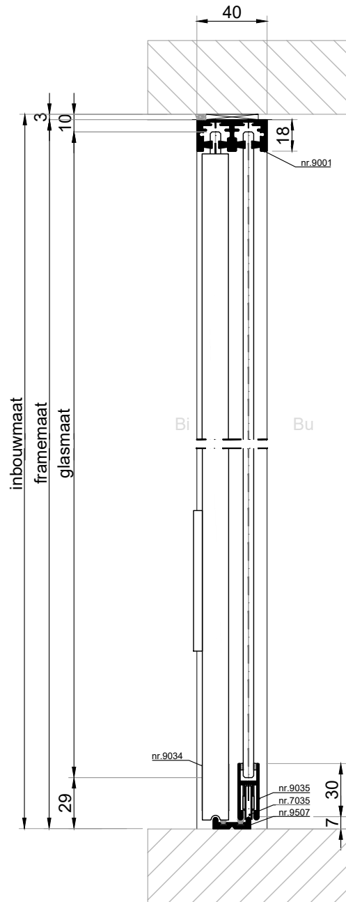
VERTICALE DOORSNEDE type HSV-3
