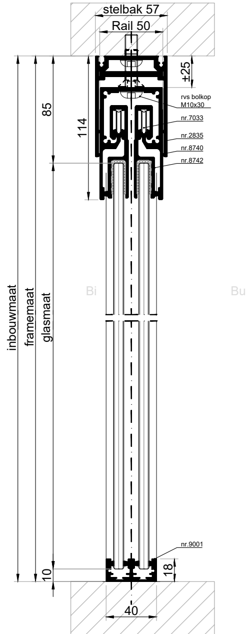
VERTICALE DOORSNEDE type ASH-2
